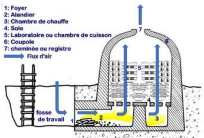
Principe de fonctionnement d'un four à faïences ancien
